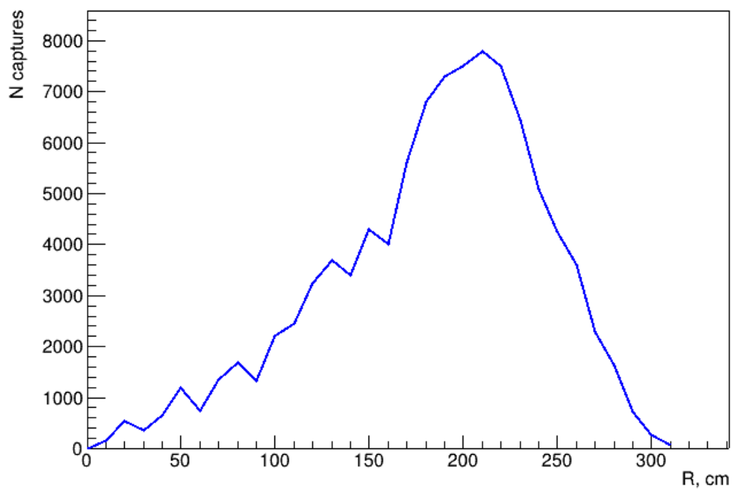
Рисунок 3.8 — Зависимость количества захватов быстрых нейтронов от радиуса
