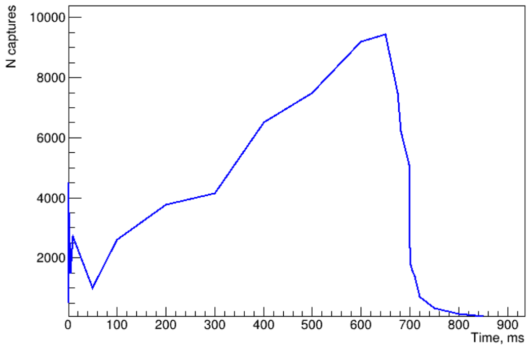
Рисунок 3.3 — Зависимость количества захватов резонансных нейтронов от времени
