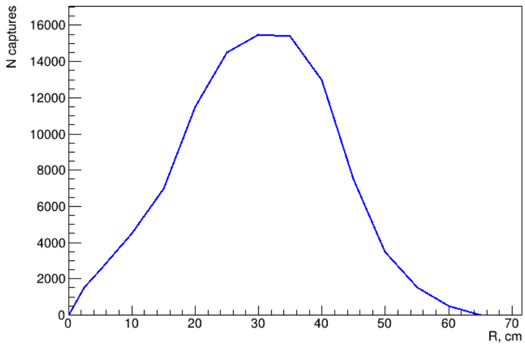
Рисунок 3.6 — Зависимость количества захватов тепловых нейтронов от радиуса
