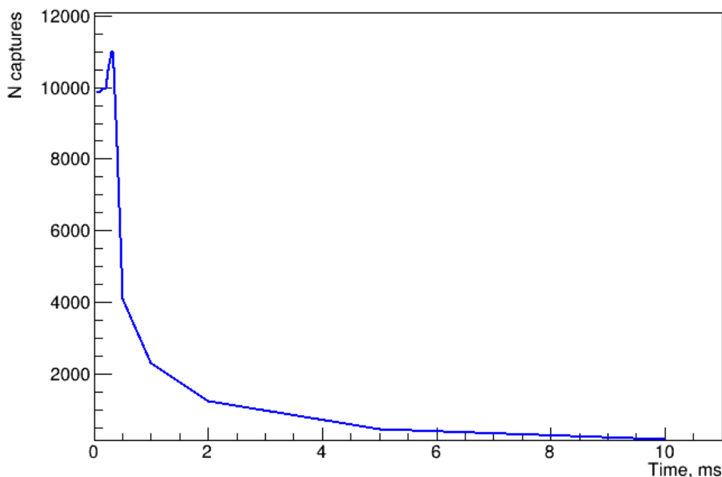
Рисунок 3.2 — Зависимость количества захватов тепловых нейтронов от времени
