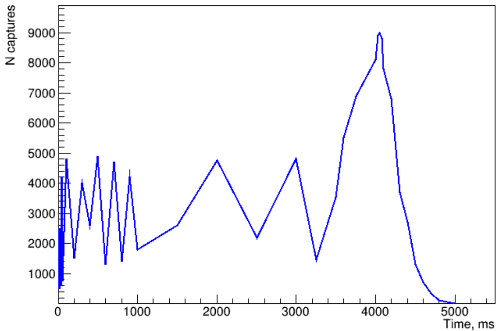
Рисунок 3.4 — Зависимость количества захватов быстрых нейтронов от времени
