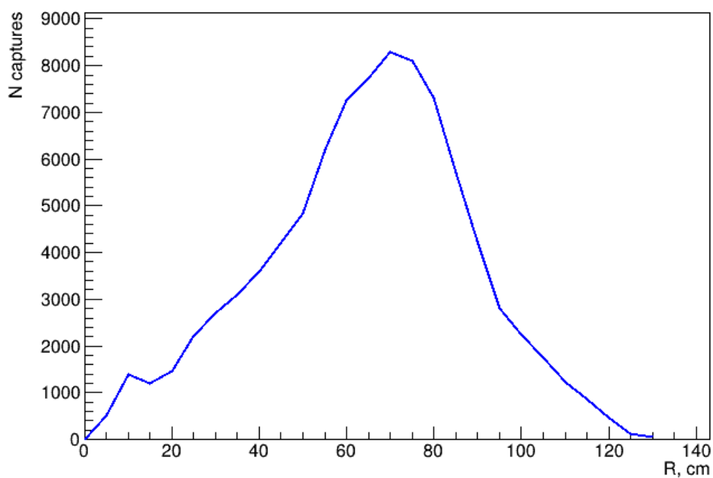
Рисунок 3.7 — Зависимость количества захватов резонансных нейтронов от радиуса
