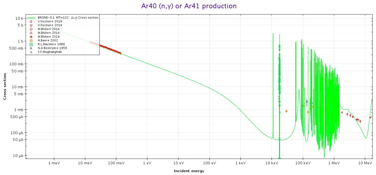
Рисунок 3.5 — Зависимость сечения захвата нейтрона от энергии его энергии
