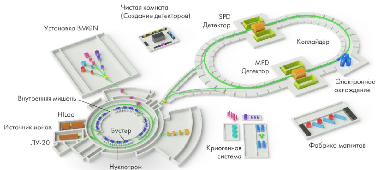
Рисунок 2 — Схема комплекса NICA
