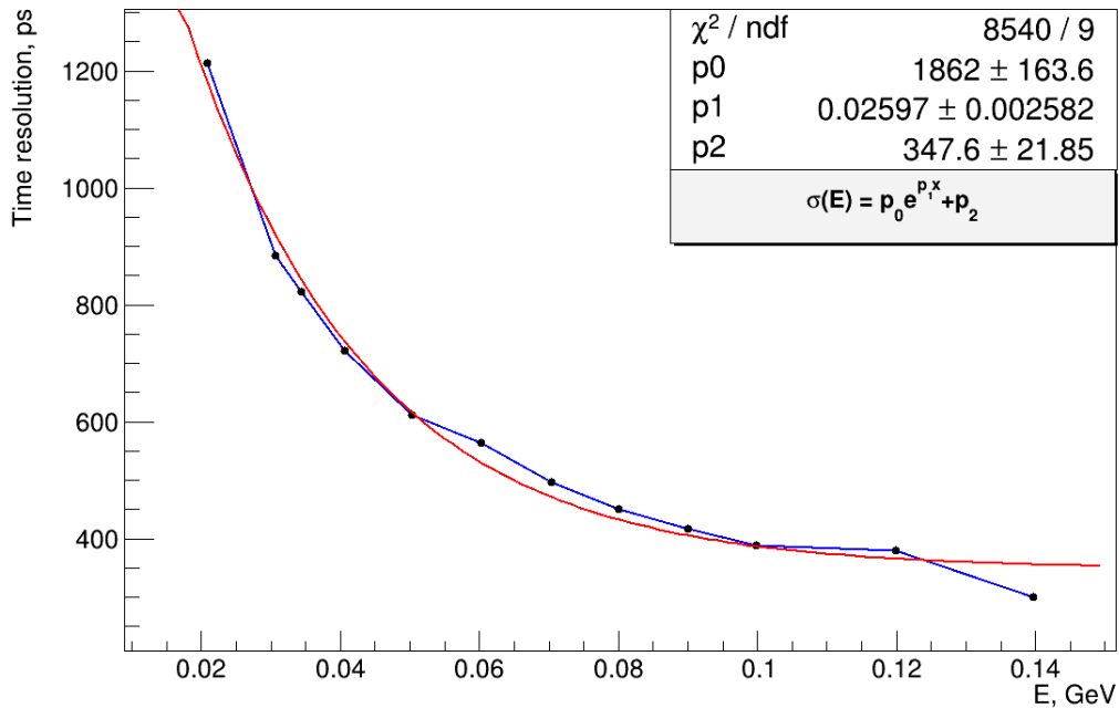
Рисунок 20 — Зависимость временного разрешения от энергии кластера
