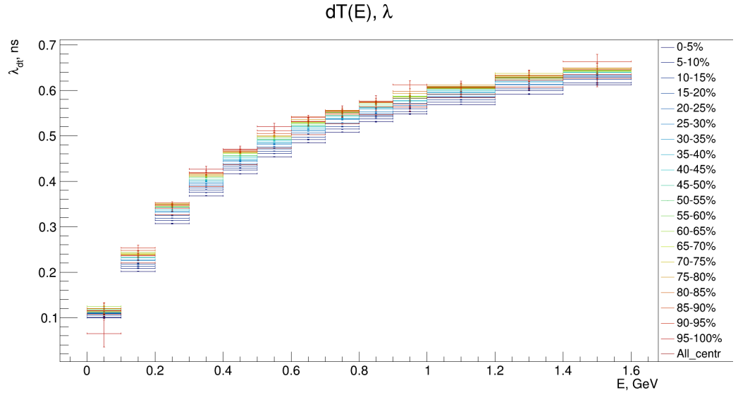
Рисунок 23 — Зависимость среднего dt от энергии кластера.
