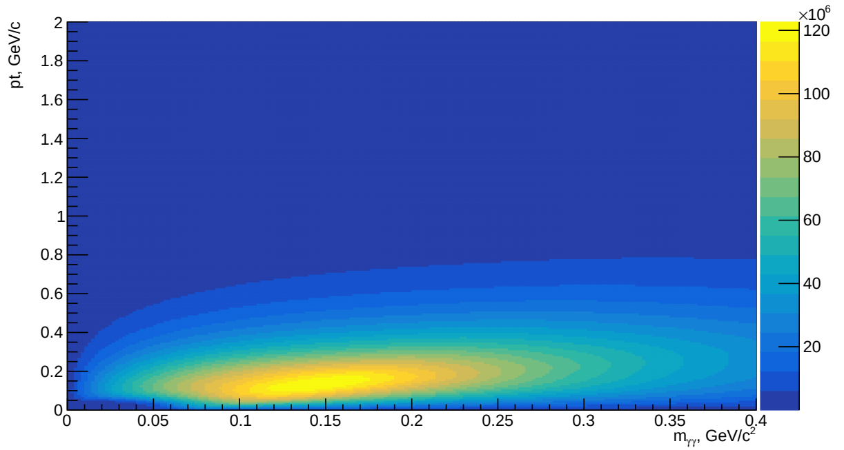
Рисунок 26 — Распределения инвариантных масс смешанных событий для диапазона центральныхностей 0-5%.
