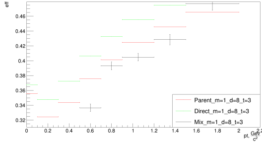
Рисунок 28 — Эффективности критериев наложенных на кластеры. Здесь Parent - кластеры, имеющие общего родителя ( \pi^0 ); Direct – кластеры, имеющие общего родителя ( \pi^0 ), вершина которого находится около вершины взаимодействия и при этом это прямой родитель кластеров; Mix - Direct кластеры, которые были получены из метода инвариантных масс.
