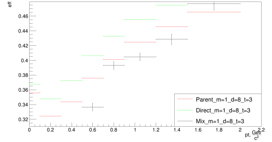
Рисунок 28 — Эффективности критериев наложенных на кластеры. Здесь Parent - кластеры, имеющие общего родителя ( \pi^0 ); Direct – кластеры, имеющие общего родителя ( \pi^0 ), вершина которого находится около вершины взаимодействия и при этом это прямой родитель кластеров; Mix - Direct кластеры, которые были получены из метода инвариантных масс.
