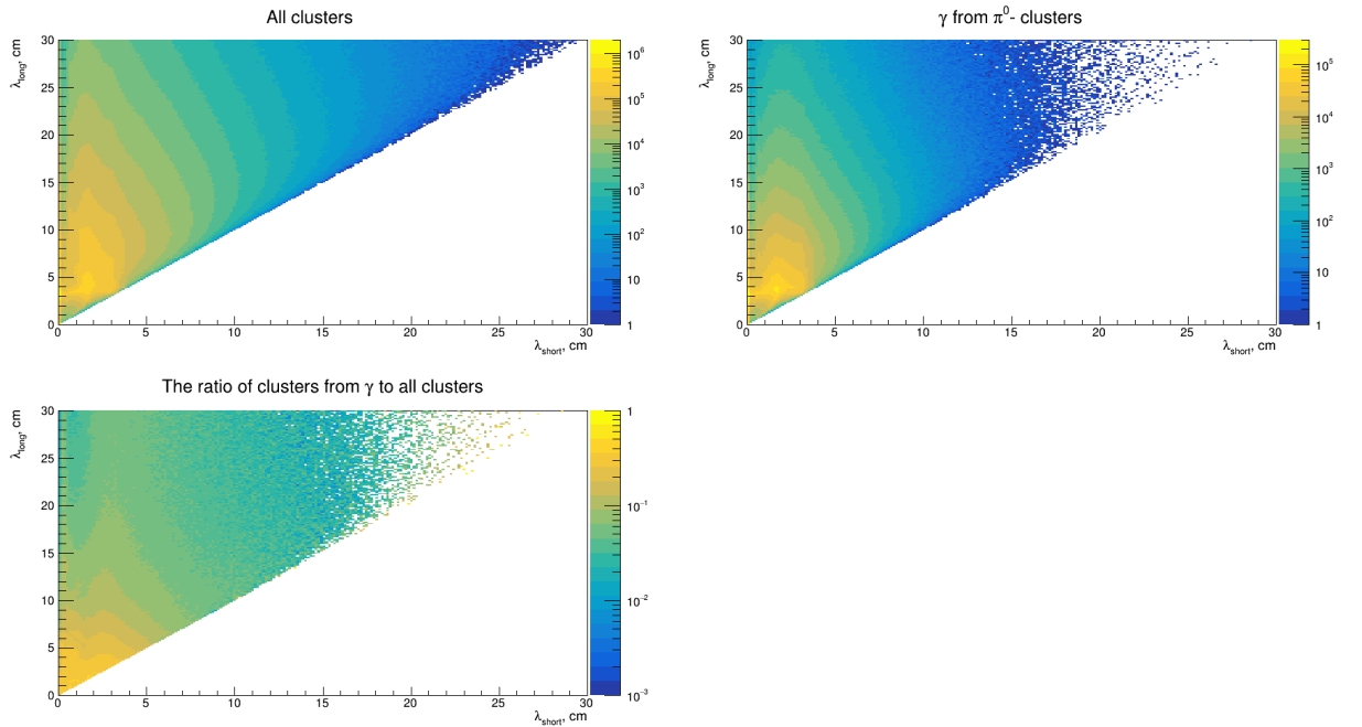
Рисунок 19 — Распределения по большой и малой дисперсии для всех центральных и энергий в диапазоне 0.4-0.5 ГэВ.
