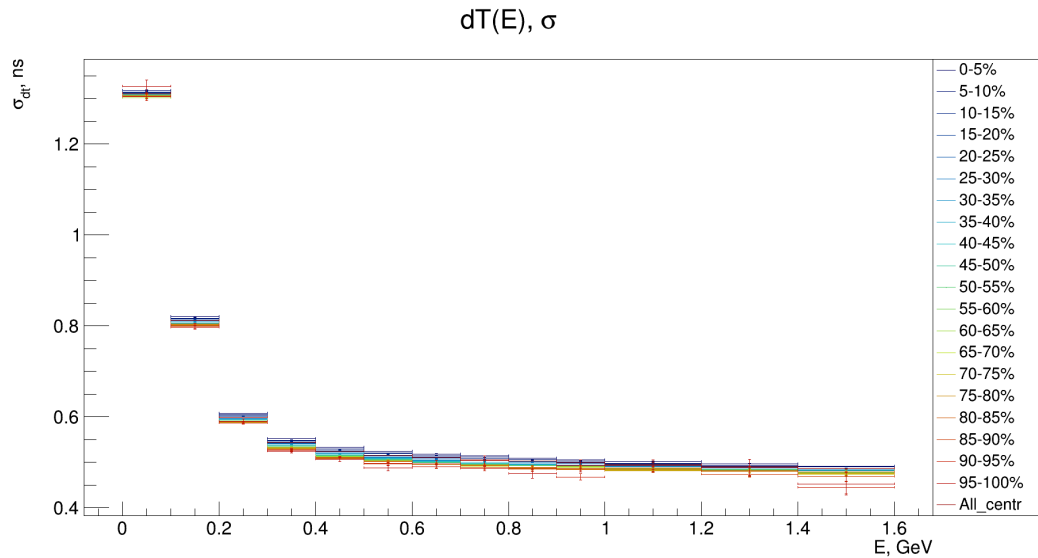
Рисунок 22 — Зависимость среднеквадратичного отклонения dt от энергии кластера.
