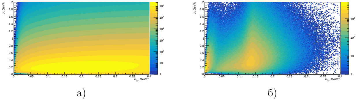
Рисунок 24 — Распределение инвариантных масс пар кластеров от поперечного импульса для диапазона центральности 0-5% для всех кластеров (а) и кластеров, порожденных \pi^0 - мезонами.
