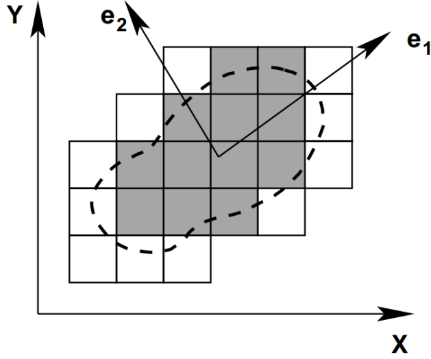
Рисунок 18 — Форма кластера
