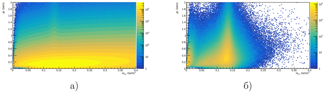
Рисунок 25 — Распределение инвариантных масс пар кластеров от поперечного импульса для диапазона центральности 50-100% для всех кластеров (а) и кластеров, порожденных \pi^0 - мезонами.
