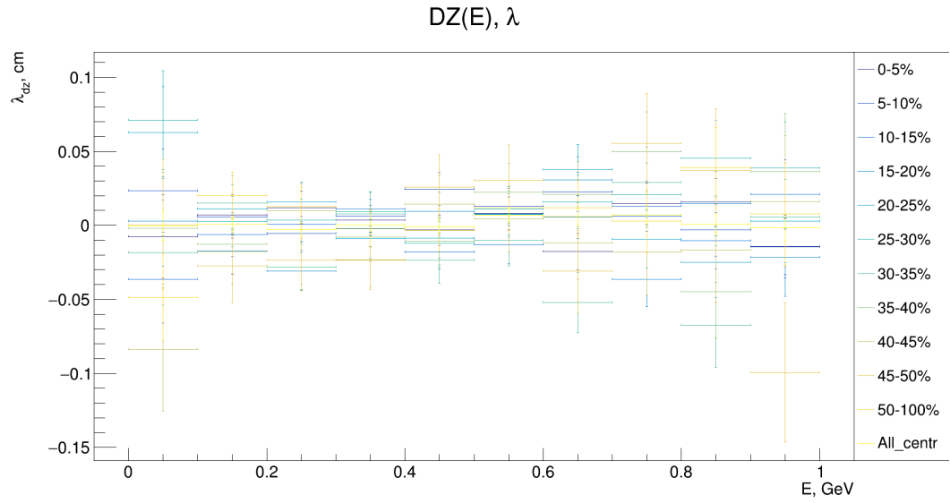
Рисунок 14 — Зависимость среднего расстояния по оси Z между заряженным кластером и ближайшим к нему треком от энергии кластера.
