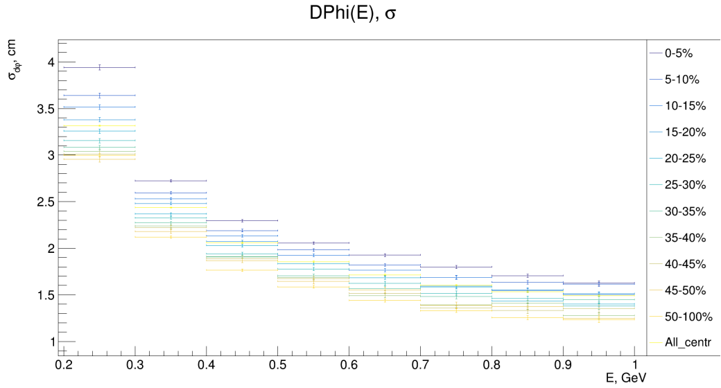
Рисунок 17 — Зависимость среднеквадратичного отклонения расстояния по оси \varphi между заряженным кластером и ближайшим к нему треком от энергии кластера.
