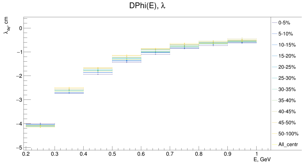
Рисунок 16 — Зависимость среднего расстояния по оси \varphi между заряженным кластером и ближайшим к нему треком от энергии кластера
