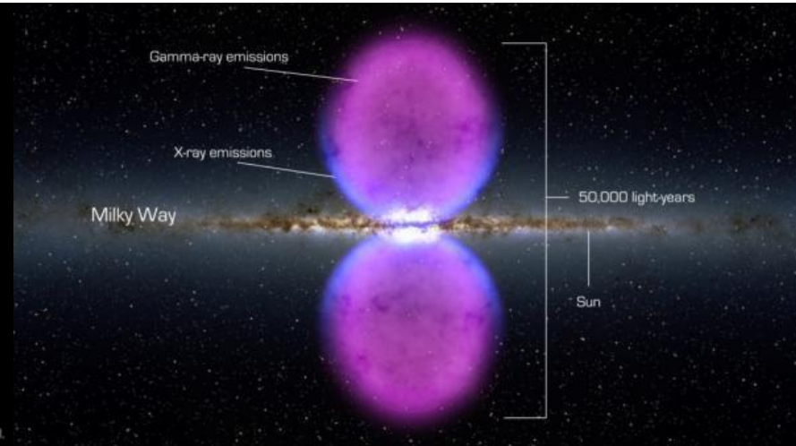
Fermi bubbles
