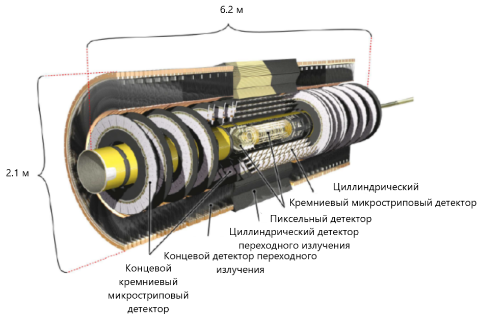
Рисунок 2.2 — Схема внутреннего детектора
