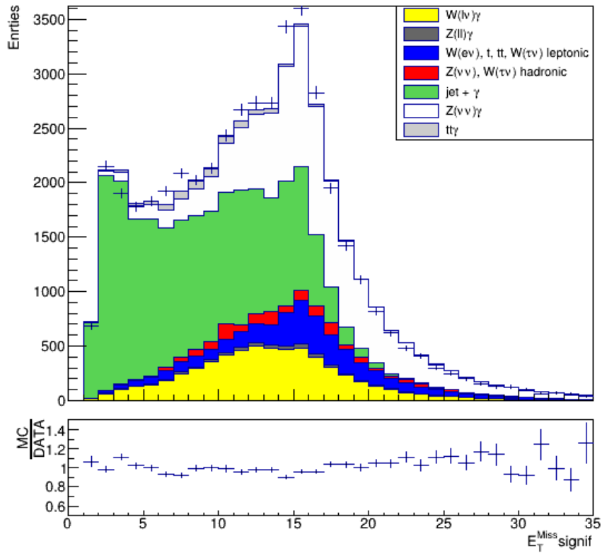
Рисунок А.1 — Распределение по E_T^{miss} значимость, построенное без отборов на переменные E_T^{miss} значимость и p_T^{SoftTerm}
