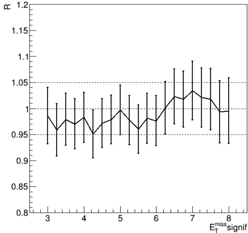
Рисунок 4.4 — График зависимости R_{data} от величины E_T^{miss} \text{ signif} , определяющей области E и F
