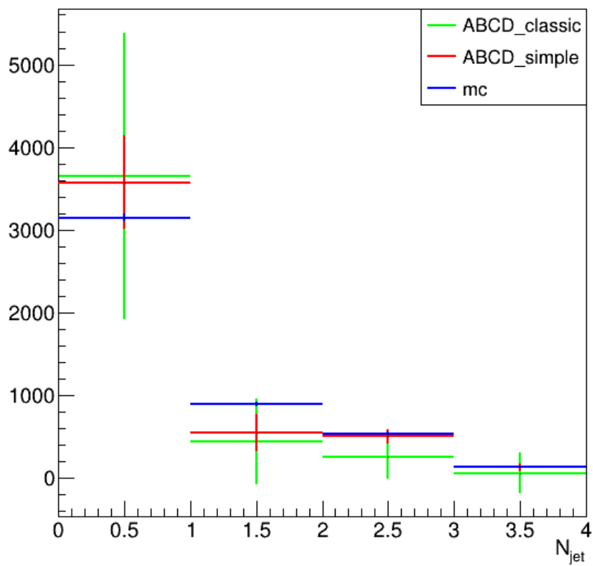
Рисунок 4.7 — Распределения фона \gamma + jet по множественности струй, полученные из Монте-Карло, классическим и упрощенным ABCD-методами
