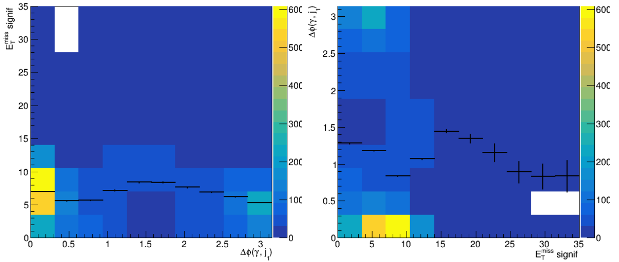
Рисунок Б.3 — Профильные гистограммы для установления корреляции по переменным E_T^{miss} значимость и \Delta\phi(\gamma, j_1) . Сняты угловые и отбор по E_T^{miss} значимость. а - профиль по \Delta\phi(\gamma, j_1) , б - профиль по E_T^{miss} значимость
