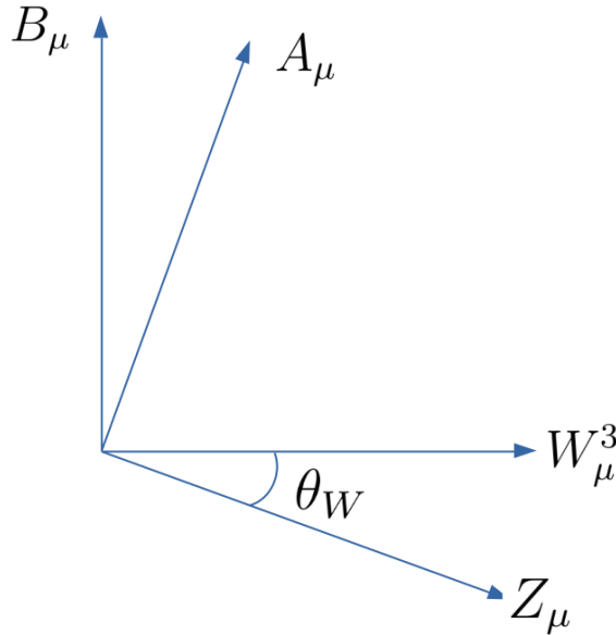
Рисунок 1.2 — Графическая интерпретация угла Вайнберга
