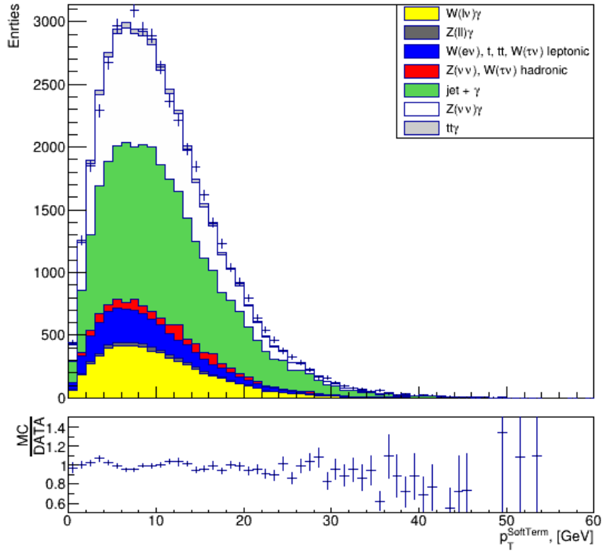
Рисунок А.2 — Распределение по p_T^{SoftTerm} , построенное без отборов на переменные E_T^{miss} значимость и p_T^{SoftTerm}
