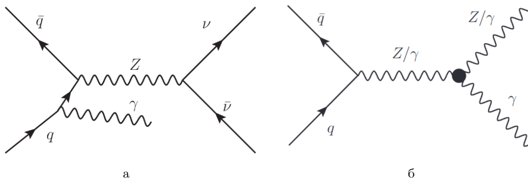
Рисунок 1 — Диаграммы Фейнмана для Z(\nu\bar{\nu})\gamma : а - испускание фотона из начального состояния, б - процесс, протекающий через трёхбозонную вершину (запрещена в СМ)
