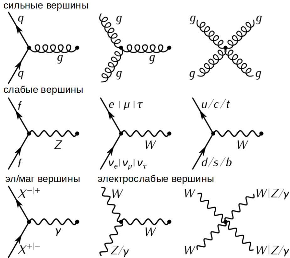
Рисунок 1.3 — Вершины в стандартной модели (вершины с бозоном Хиггса не указаны)
