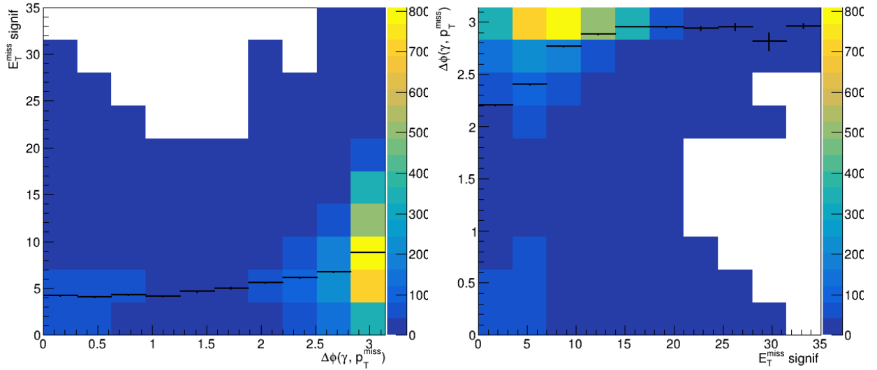
Рисунок Б.2 — Профильные гистограммы для установления корреляции по переменным E_T^{miss} значимость и \Delta\phi(\gamma, p_T^{miss}) . Сняты угловые отборы и отбор по E_T^{miss} значимость. а - профиль по \Delta\phi(\gamma, p_T^{miss}) , б - профиль по E_T^{miss} значимость
