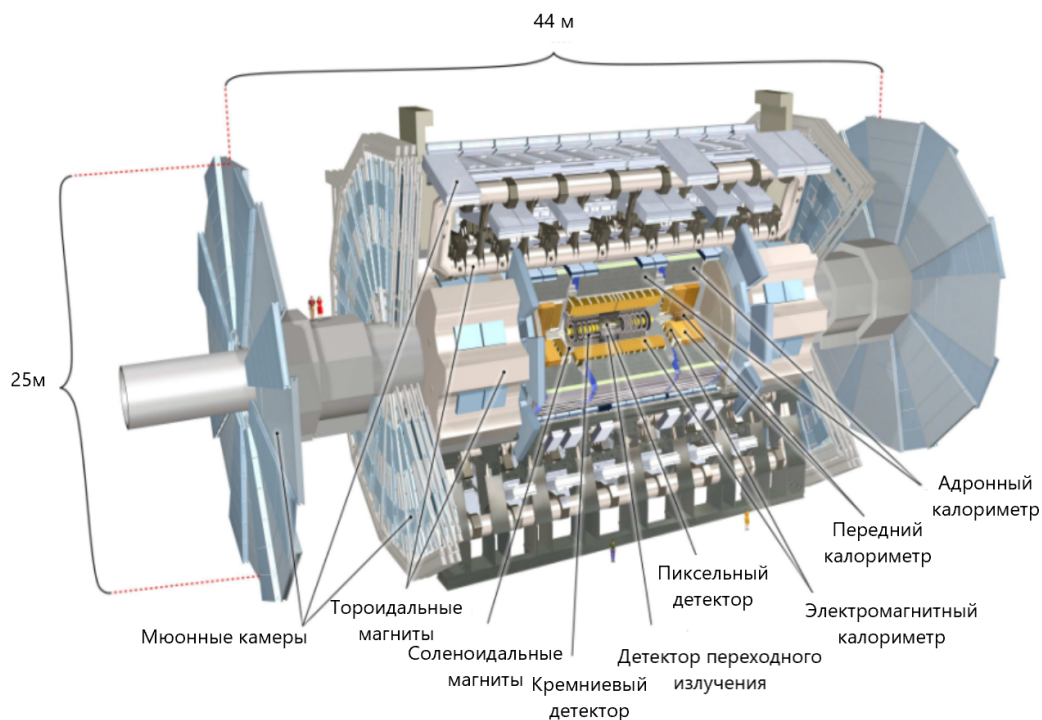
Рисунок 2.1 — Схема детектора ATLAS
