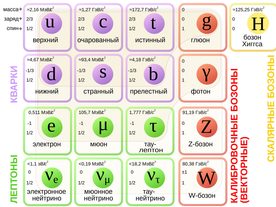
Рисунок 1.1 — Стандартная модель
