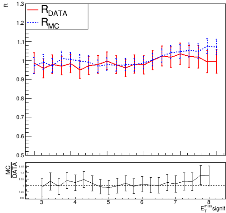
Рисунок 4.5 — График зависимости R_{data} и R_{mc} от величины E_T^{miss} значимость, определяющей области E и F
