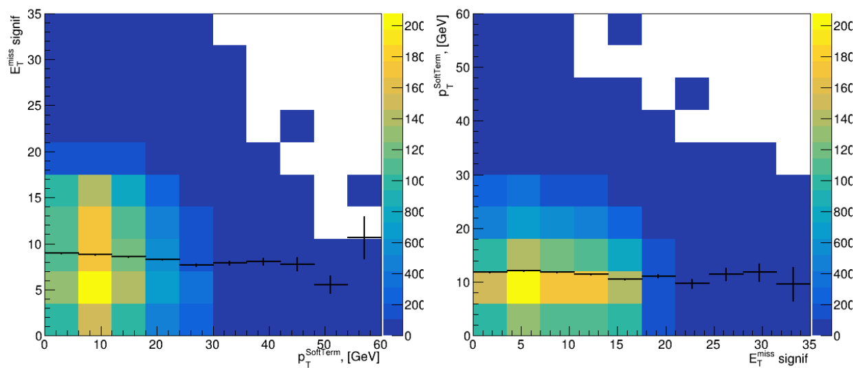
Рисунок Б.1 — Профильные гистограммы для установления корреляции по переменным E_T^{miss} значимость и p_T^{SoftTerm} . Сняты отборы только по этим переменным. а - профиль по p_T^{SoftTerm} , б - профиль по E_T^{miss} значимость
