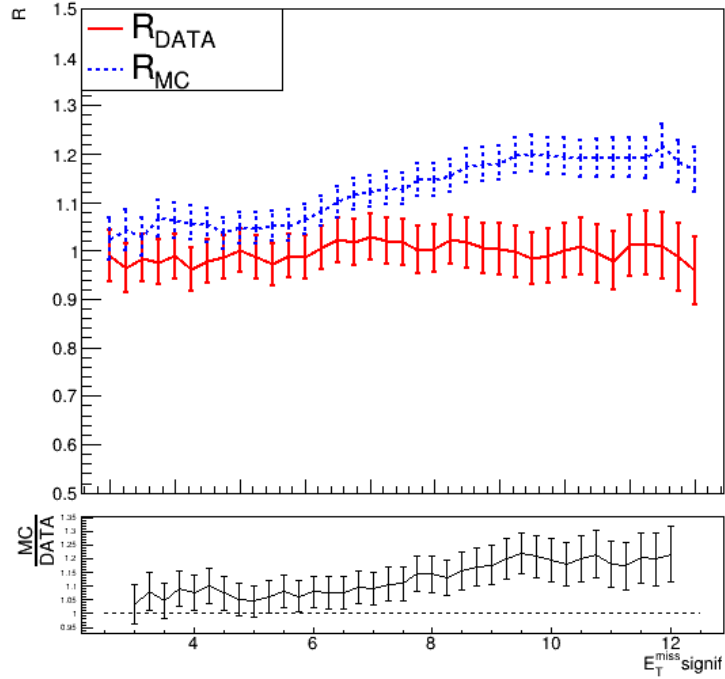
Рисунок 4.6 — График зависимости R_{data} и R_{mc} от величины E_T^{miss} значимость, определяющей области E и F. Отбор по E_T^{miss} значимость поднят с 11 до 15
