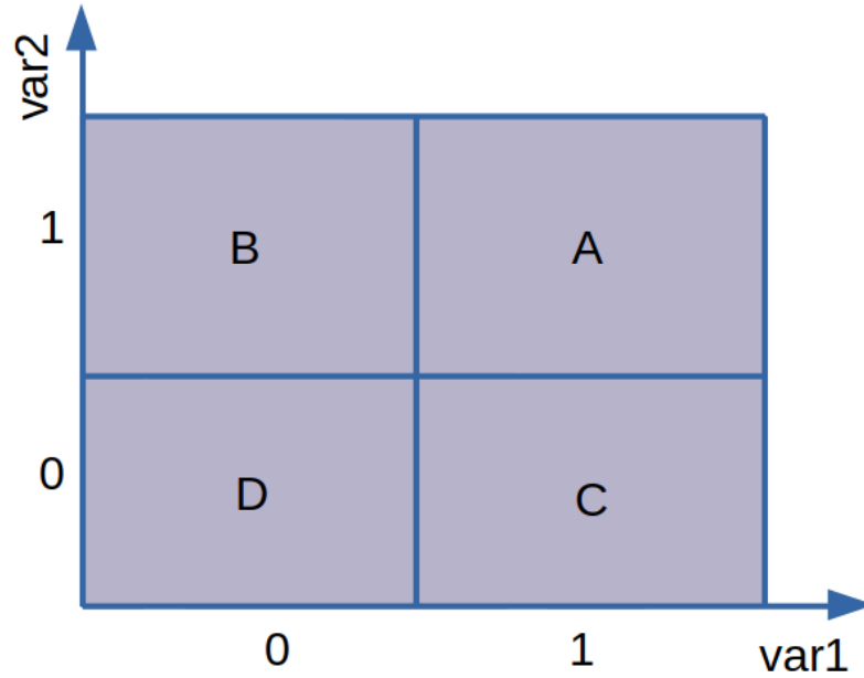
Рисунок 4.2 — Области, рассматриваемые в ABCD-методе с использованием логических конфигураций
