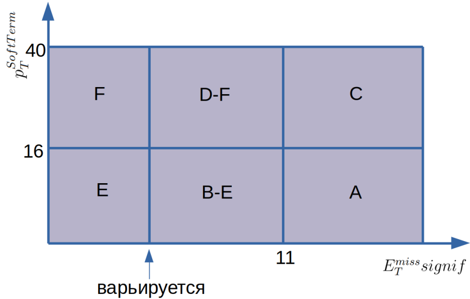
Рисунок 4.3 — Области, рассматриваемые в расширенном ABCD методе оценки R из данных
