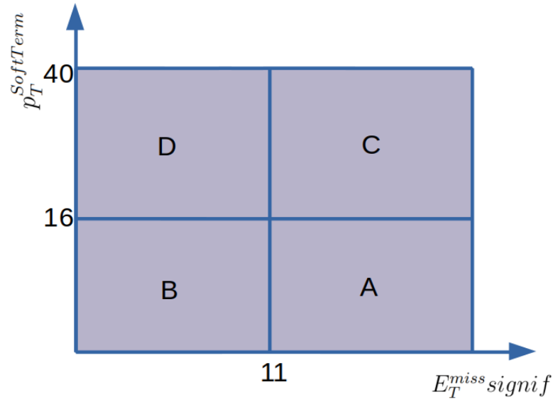
Рисунок 4.1 — Области, рассматриваемые в ABCD методе оценки фона \gamma + jet
