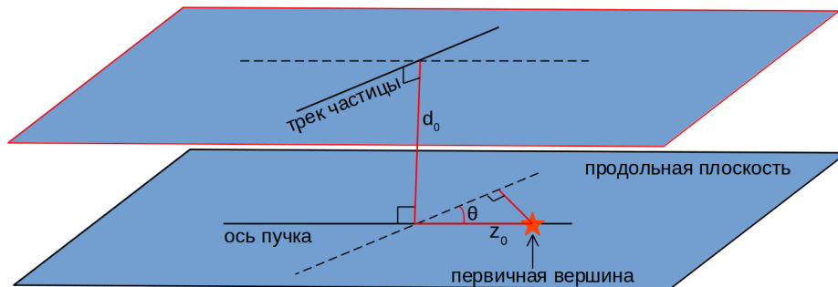
Рисунок 3.1 — Прицельные параметры d_0 и z_0
