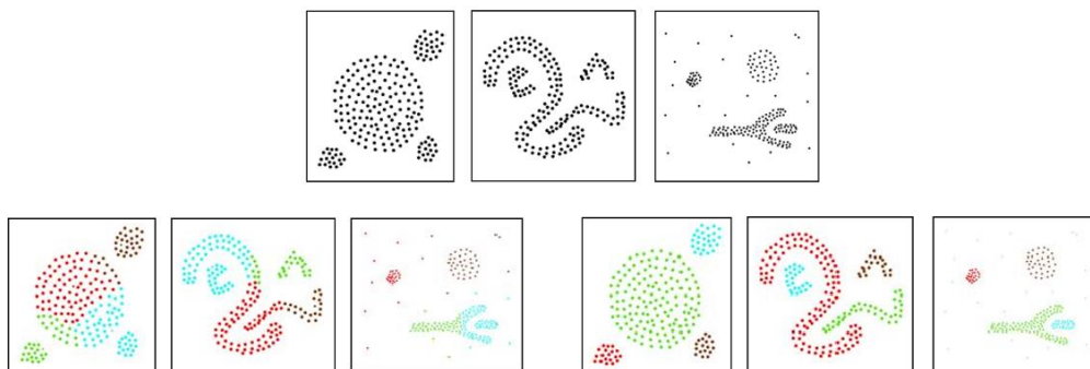
Рис. 4 Иллюстрация работы алгоритмов кластеризации. Сверху изображен оригинальный набор точек. Слева снизу – результат работы алгоритма CLARANS. Справа снизу – алгоритма DBSCAN.
