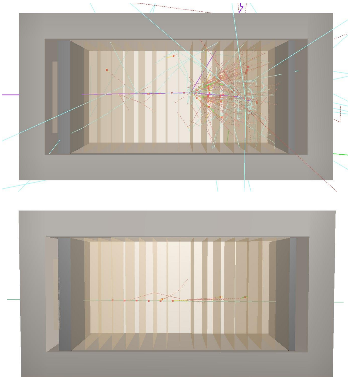
Рис. 7 Прохождения протона и мюона с энергией 10 ГэВ через прототип. Сверху – протон, снизу – мюон.
