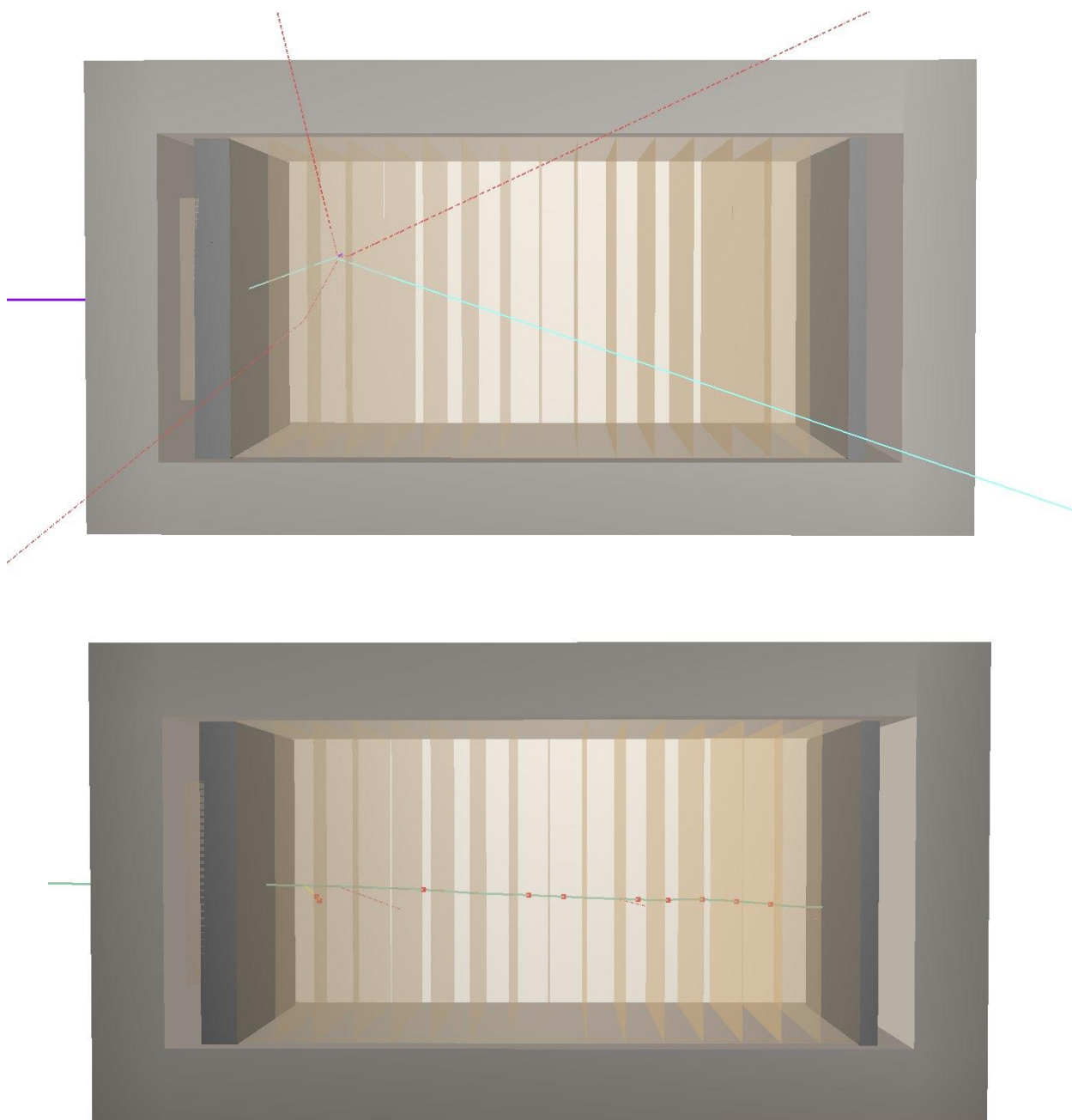
Рис. 6 Прохождения протона и мюона с энергией 1 ГэВ через прототип. Сверху – протон, снизу – мюон.
