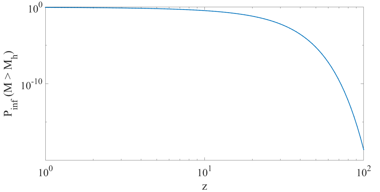
Рисунок 4 — График зависимости доли материи с массой большей, чем M_h , P_{\text{inf}}(M > M_h) от красного смещения z .
