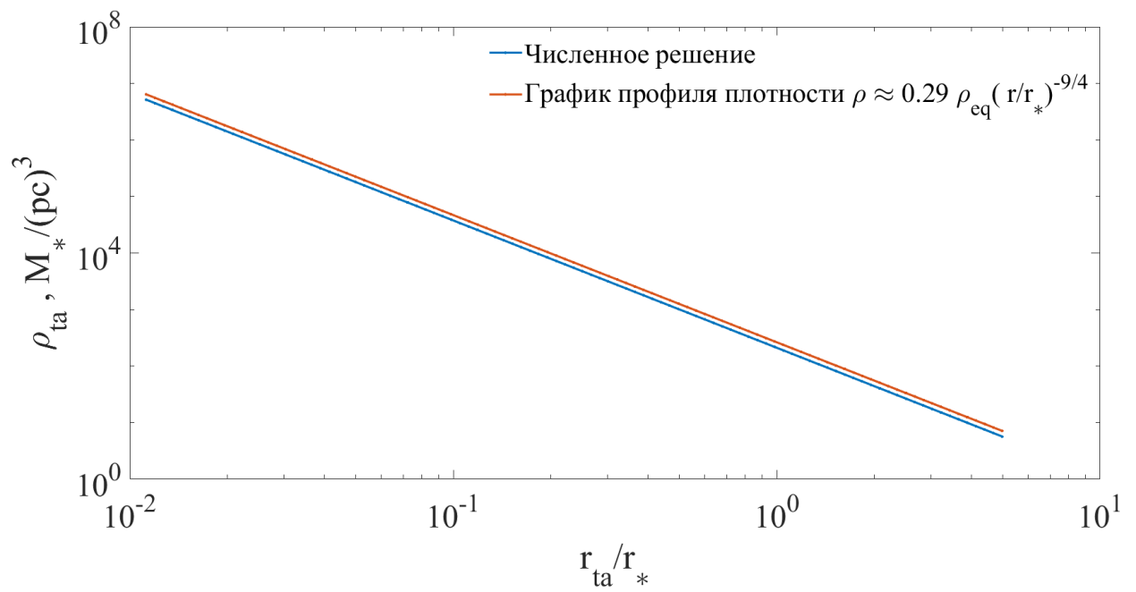
Рисунок 3 — Профиль плотности сферической оболочки материи, масштабированный как \rho(r/r_*) , где r_* = (M_{PBH}/\rho_{\text{eq}})^{1/3} . Синей пунктирной линией обозначена зависимость, полученная при численном решении 3.2, красной — зависимость, полученная при аналитическом решении.
