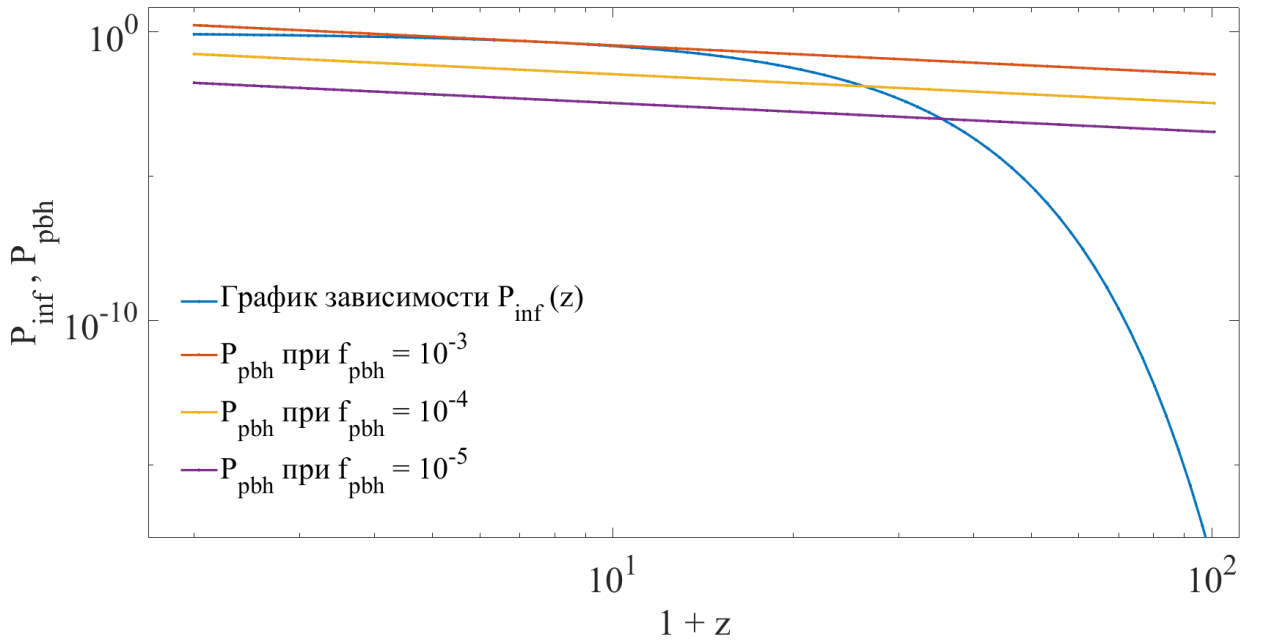
Рисунок 6 — Графическое решение уравнения (20). Точка пересечения синей и красной пунктирных линий показывает момент остановки роста гало вокруг первичной черной дыры при f_{PBH} = 10^{-3} ; синей и желтой пунктирных линий — момент остановки роста гало при f_{PBH} = 10^{-4} ; синей и фиолетовой — момент остановки роста гало при f_{PBH} = 10^{-5} .
