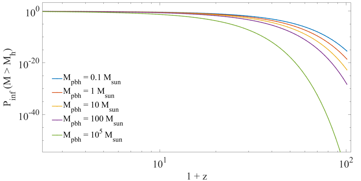
Рисунок 5 — Графики зависимости доли материи с массой большей, чем M_h , P_{\text{inf}}(M > M_h) от красного смещения 1+z для различных масс M_{PBH} .
