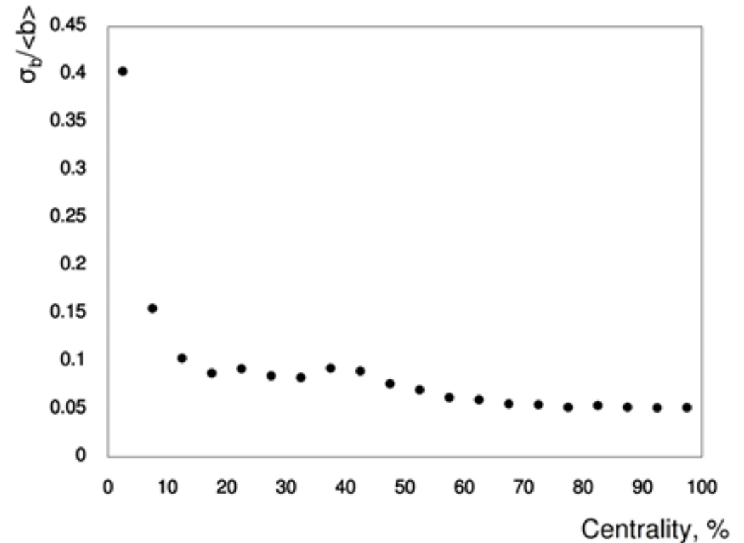
LAQGSM
