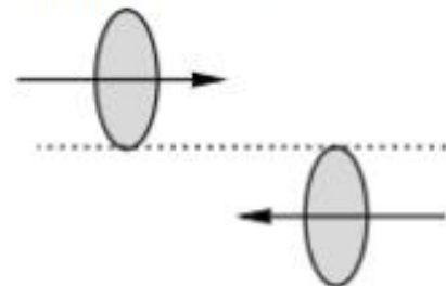
Периферическое столкновение
