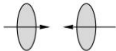
Центральное столкновение
