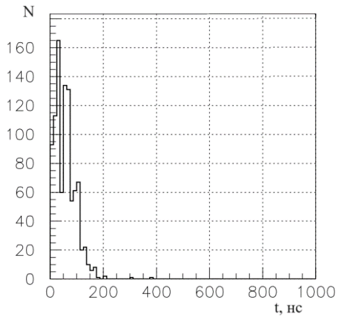
Рисунок 4.3 — Распределение времени срабатывания счетчиков в мюонном событии
