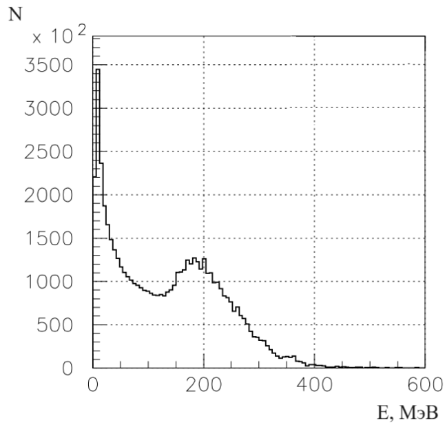
Рисунок 4.1 — Распределение энерговыделений в одном счетчике
