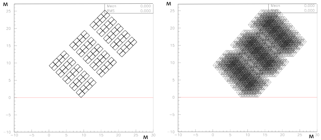
Рисунок 4.4 — Проекция счётчиков установки LVD: слева — \varphi = 45^\circ , \theta = 0^\circ ; справа — \varphi = 45^\circ , \theta = 30^\circ
