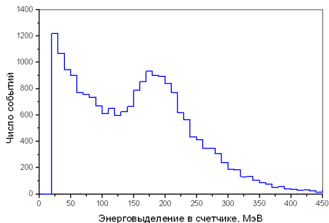
Рисунок 2.6 — Энерговыделение в счетчике при прохождении почти горизонтальных мюонов
