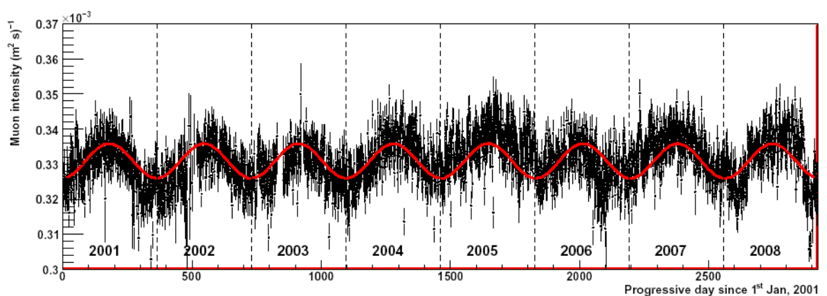
Рисунок 2.8 — Вариация интенсивности потока мюонов
