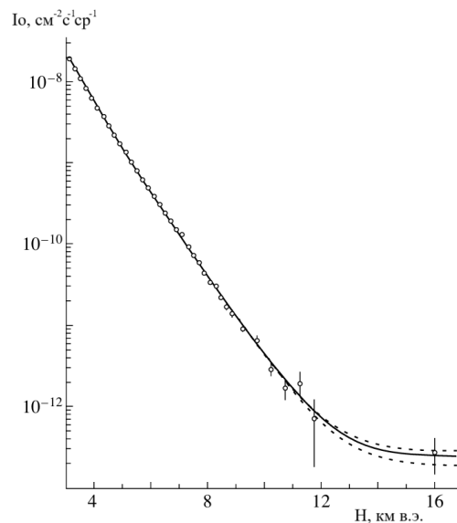
Рисунок 2.7 — Интенсивность вертикальных мюонов как функция глубины
