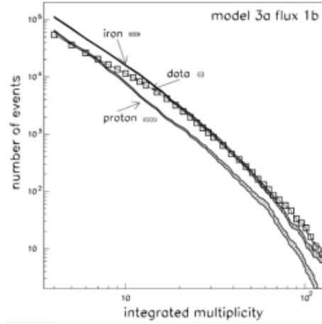
Рисунок 1.3 — Интегральное распределение событий по множественности мюонов в эксперименте DELPHI
