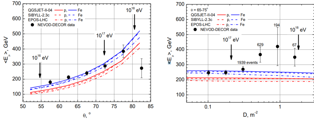
Рисунок 1.4 — Зависимость средней энергии мюонов в группах мюонов от зенитного угла (рисунок слева) и локальной плотности мюонов для зенитных углов \theta = 65^\circ\text{--}75^\circ (рисунок справа). Точки — полученные данные; кривые — ожидаемые зависимости для групп мюонов ШАЛ, образованных первичными протонами (сплошная) и ядрами железа (штриховая). Стрелками указаны характерные энергии первичных частиц космических лучей
