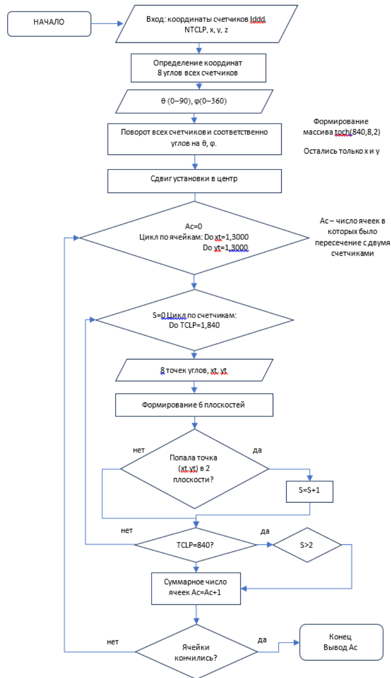
Рисунок 4.5 — Блок-схема программы вычисления аксептанса детектора
