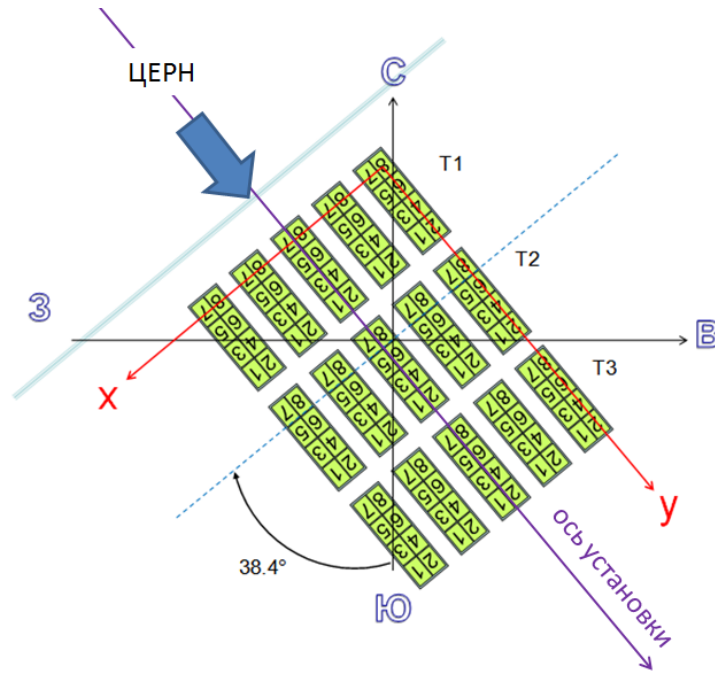
Рисунок 2.2 — Ориентация установки LVD по сторонам света
