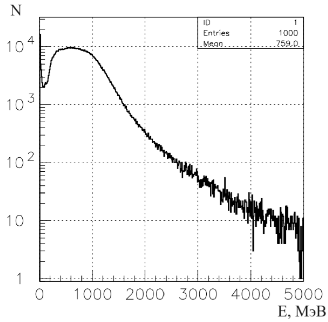
Рисунок 4.2 — Распределение суммарных энерговыделений в мюонном событии
