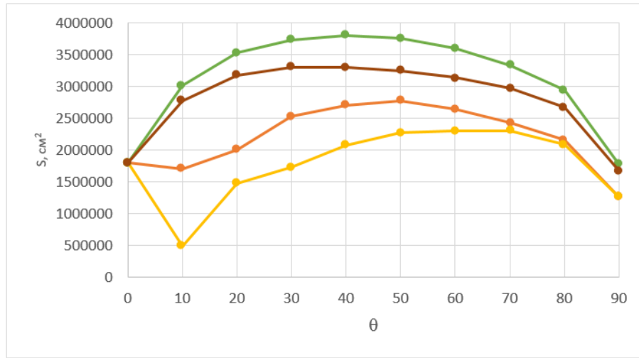
Рисунок 4.8 — Зависимость площади регистрации установки от угла \theta при фиксированных углах \varphi . Верхние кривые соответствуют \varphi = 0^\circ (с отбором N > 2 и без отбора N > 1 ), нижние кривые — \varphi = 45^\circ (с отбором и без)
