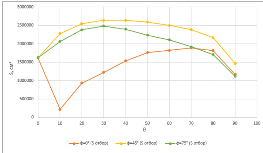
Рисунок 4.10 — Зависимость площади регистрации установки от угла \theta при фиксированных углах \varphi
