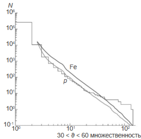
Рисунок 1.2 — Интегральное распределение событий по множественности мюонов в эксперименте ALEPH
