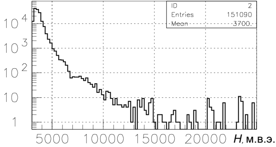
Рисунок 3.9 — Распределение числа событий по глубинам
