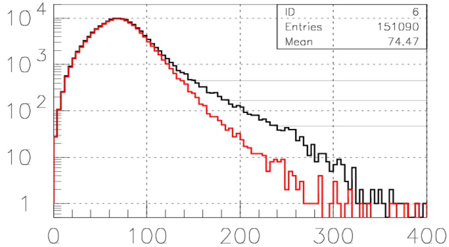
Рисунок 3.8 — Распределение событий по E/(k_m N) . Красная гистограмма — без учёта мюонов, реконструированных как одиночные мюоны
