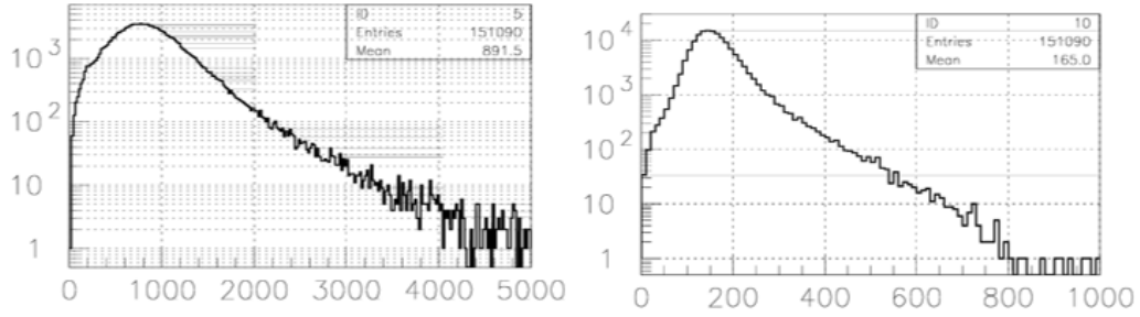
Рисунок 3.7 — Распределение событий по (E/k_m) (слева) и по (E/N) (справа)
