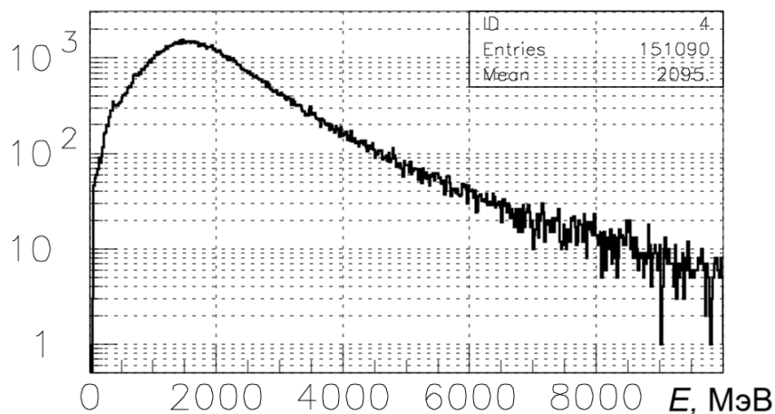
Рисунок 3.3 — Распределение по суммарному энергосвечению, реконструированных мюонных групп в детекторе
