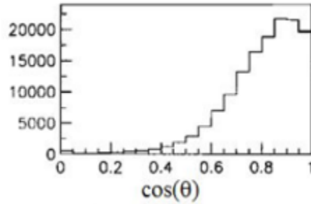
Рисунок 2.4 — Зависимость интенсивности от угла прихода мюонов
