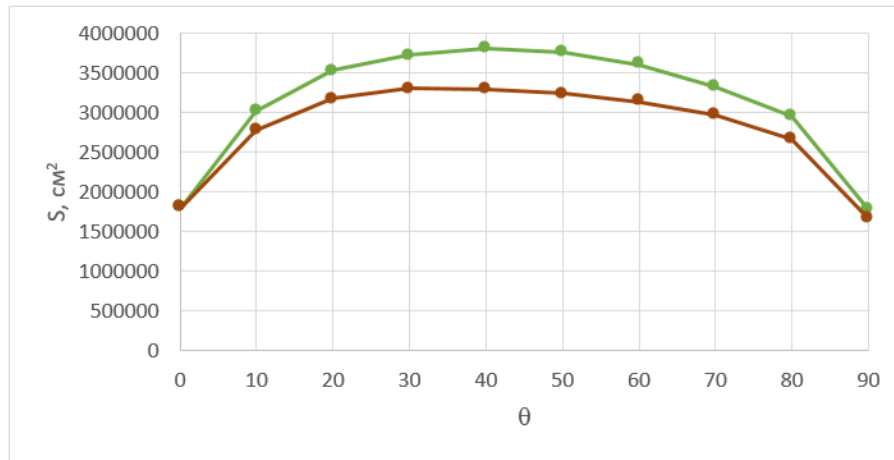
Рисунок 4.7 — Зависимость площади регистрации установки от угла \theta при фиксированном угле \varphi = 0^\circ . Верхняя кривая — без отбора, нижняя — с отбором
