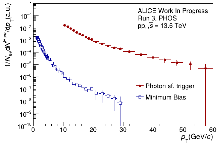
Рисунок 4.6 — Значения относительного выхода \pi^0 для различных триггеров.
