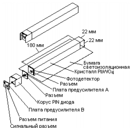
Рисунок 3.9 — Схема детектирующего элемента PHOS
