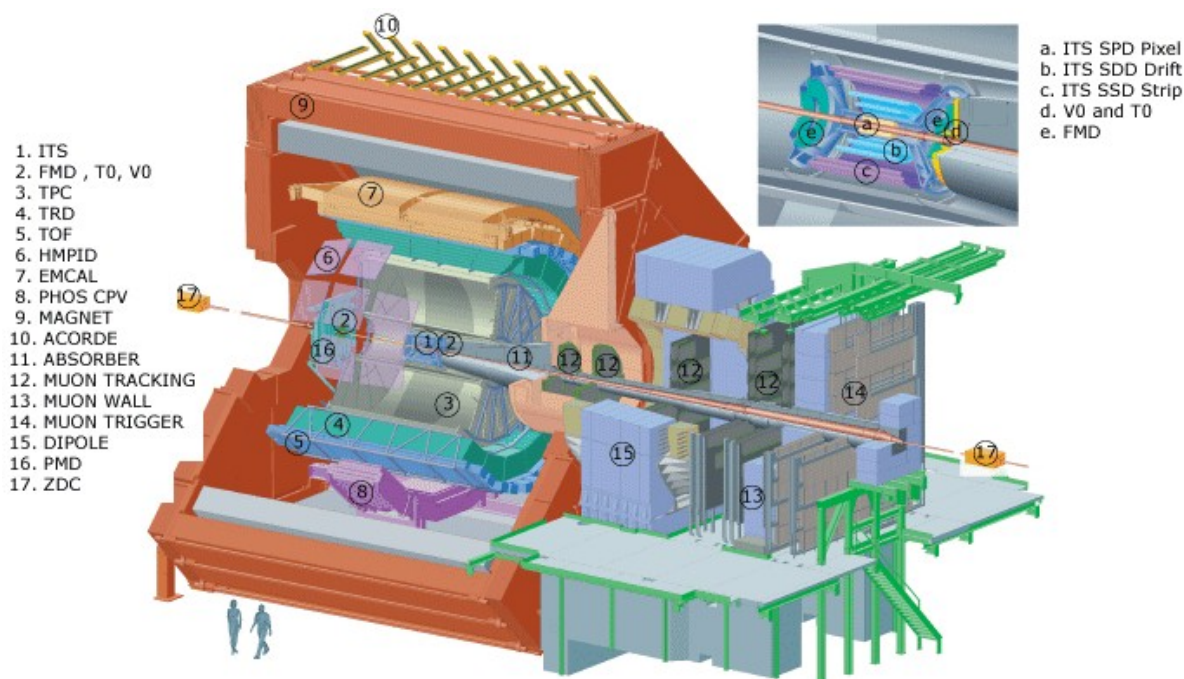
Рисунок 3.7 — Схема детектора ALICE
