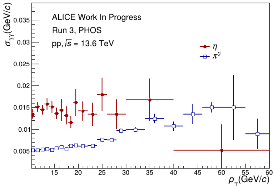
Рисунок 4.5 — Значения \sigma_{\gamma\gamma} для различных периодов в зависимости от p_T бина
