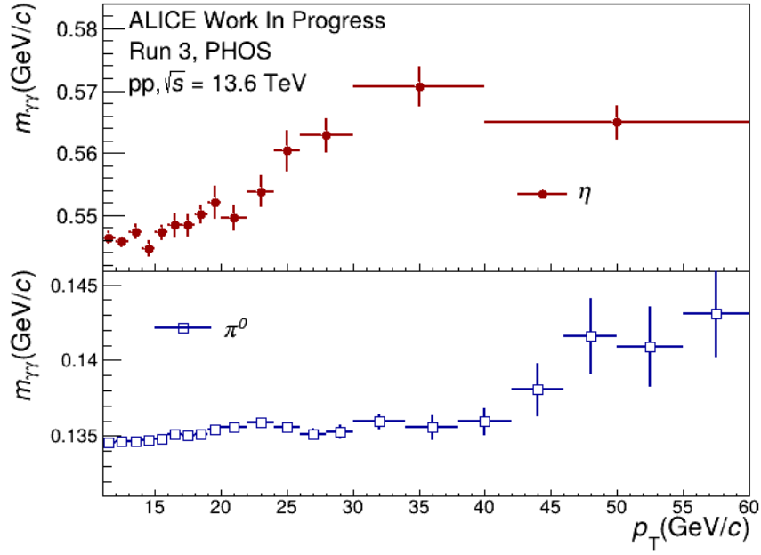
Рисунок 4.4 — Значения m_{\gamma\gamma} для различных периодов в зависимости от p_T бина
