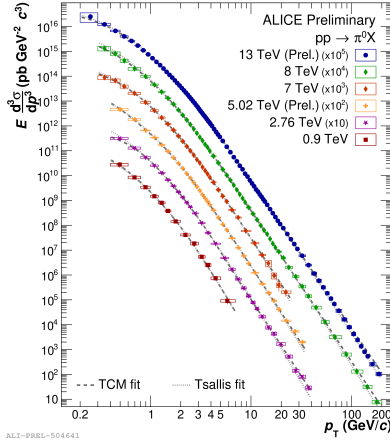
Рисунок 1.1 — Инвариантные спектры \pi^0 -мезонов в pp -столкновениях при различных энергиях
