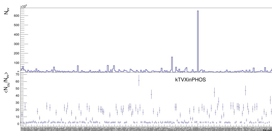
Рисунок 4.7 — QA для сенса набора данных за 2023 год
