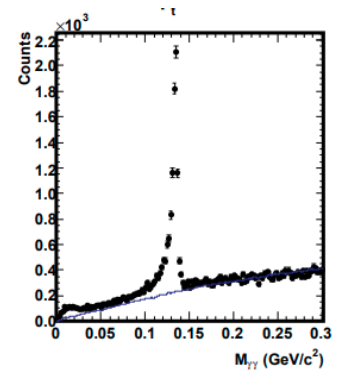
Рисунок 2.7 — Сигнальное распределение для \pi^0 -мезонов с применением конверсии
