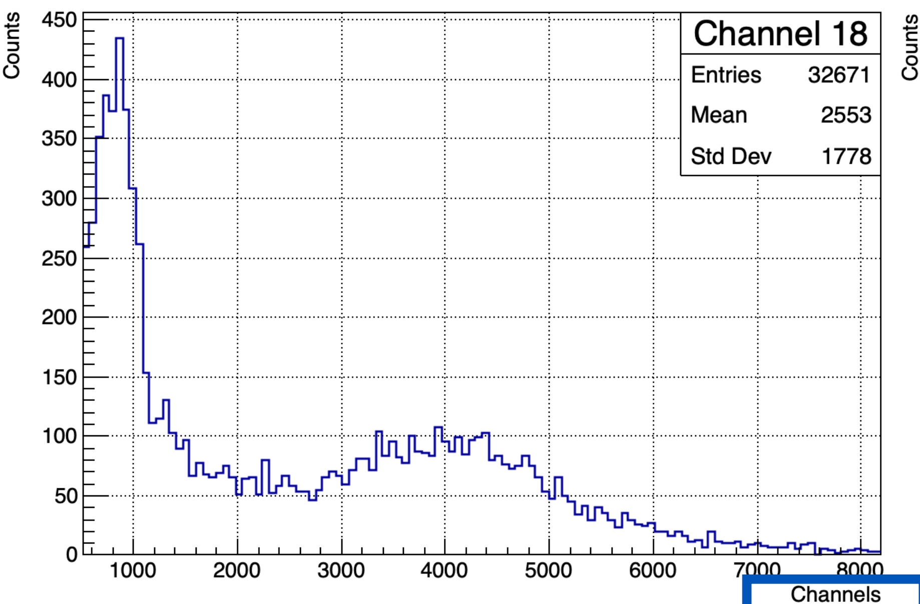
Спектр энергетических потерь космических мюонов
