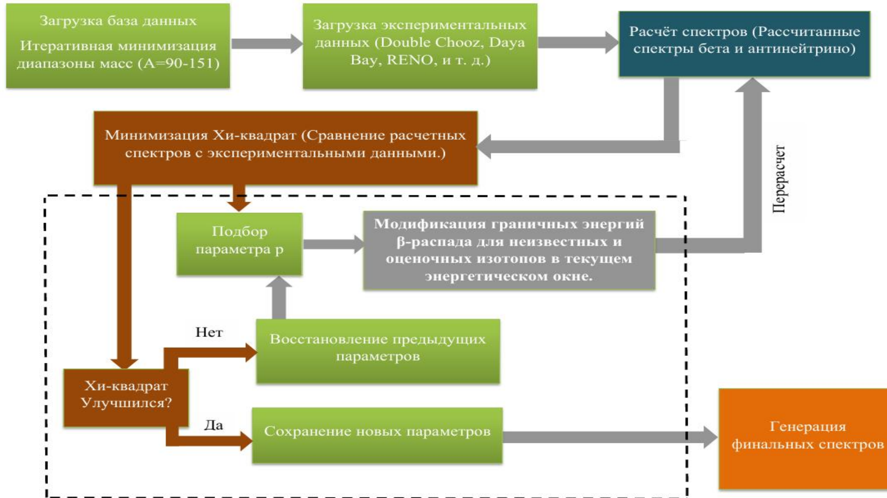
Рис 3. Блок-схема реализации метода суммирования на C++ и итеративного алгоритма для подгонки антинейтрино с минимизацией \chi^2 .
