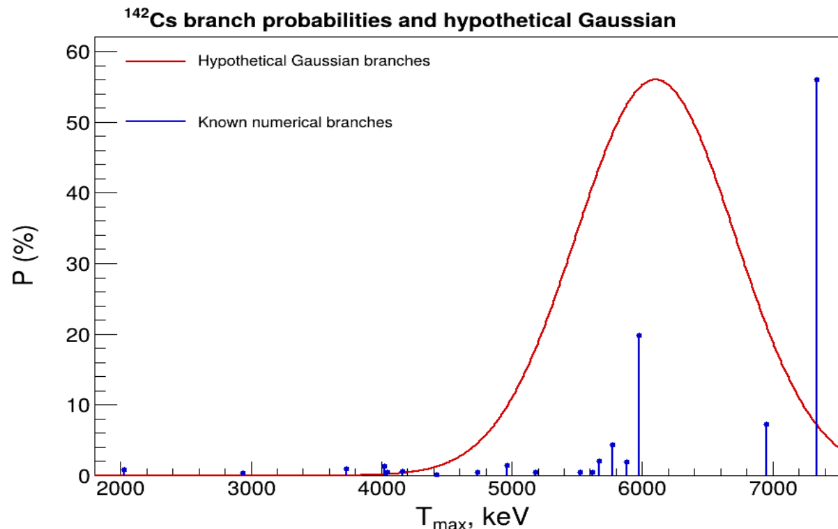
Рис.2: Вероятности ветвления для цезия ( ^{142}\text{Cs} ) и предложенных гипотетических ветвей.
