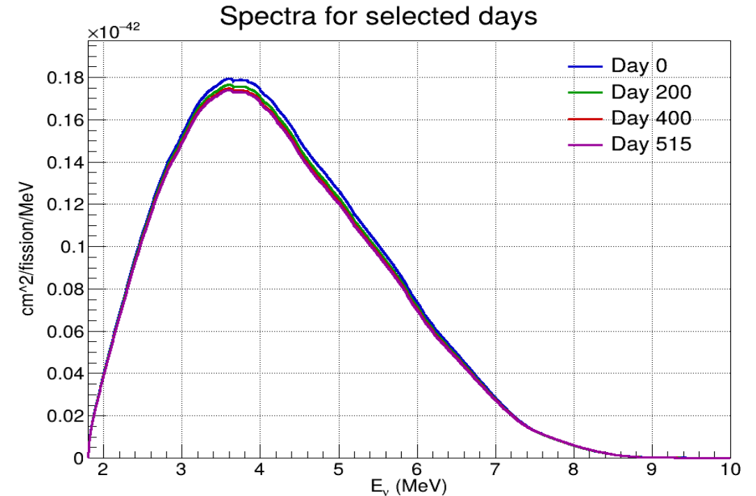
Рис.6: Изменение формы спектра антинейтрино во время кампании
