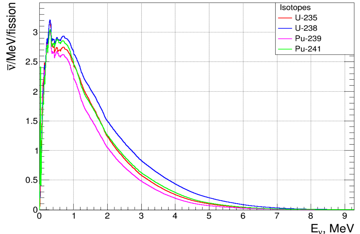
Рис.4: Спектры антинейтрино, рассчитанные с использованием экспериментальных данных Daya Bay
