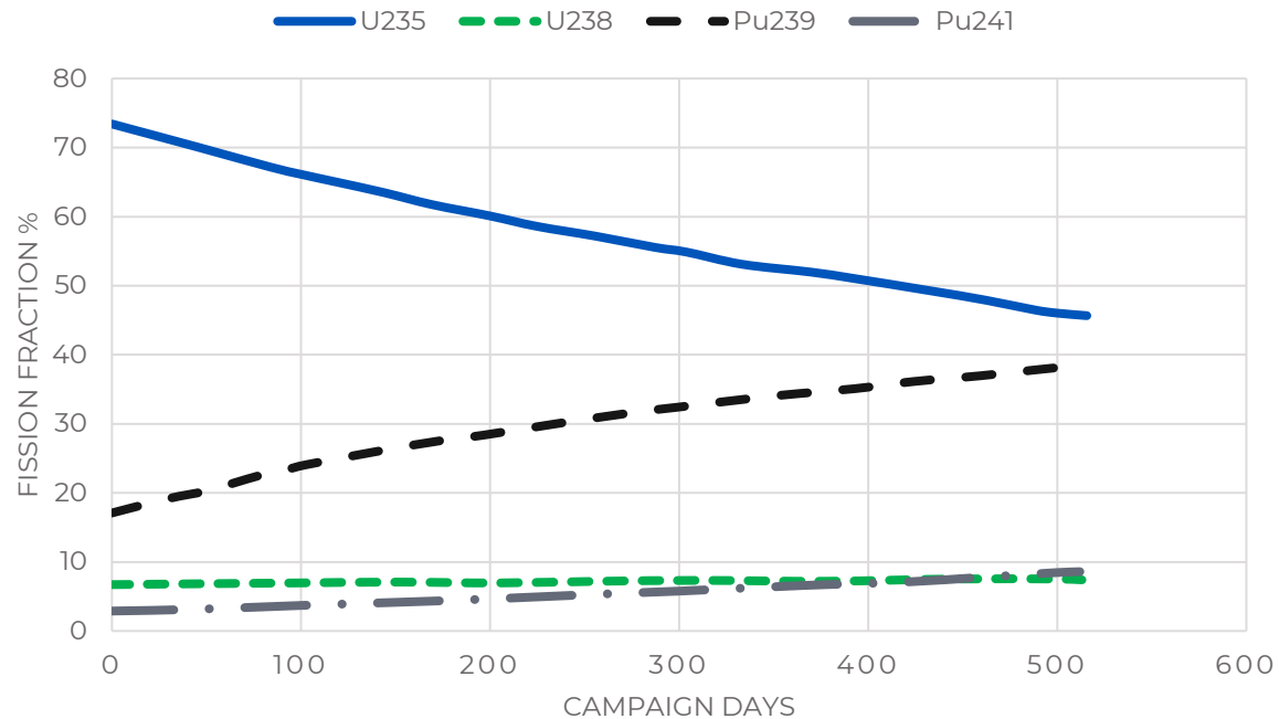
Рис.5: Доля деления во время реакторной кампании
