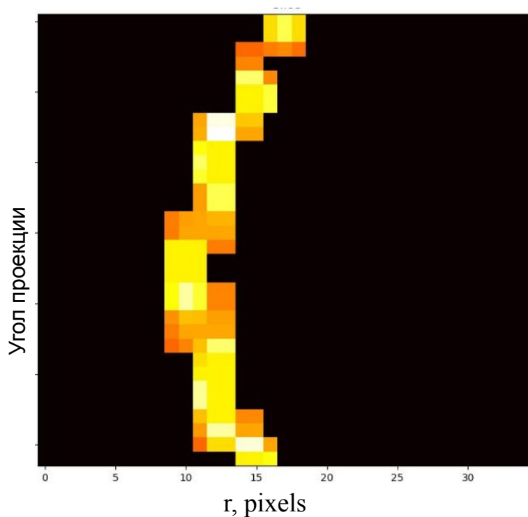
а) синограмма
