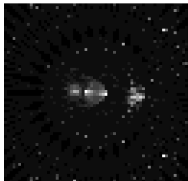
5 итераций
