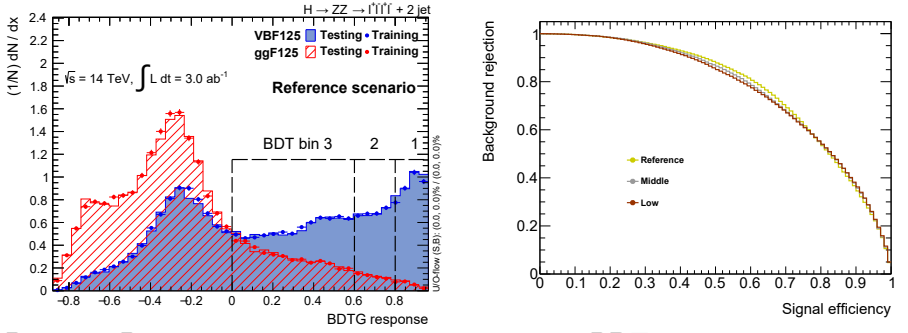
Рис. 9 — Распределение по отклику алгоритма BDT для сценария покрытия трековой системы “Reference (слева) и кривые ошибок для всех трёх рассматриваемых сценариев (справа) [6].
