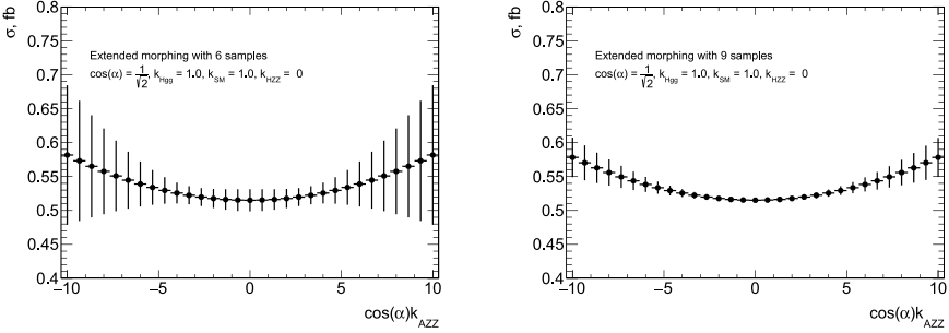
Рис. 3 — Реконструированное распределение полного сечения процесса pp \rightarrow H \rightarrow ZZ^* \rightarrow 4l как функция произведения \cos(\alpha)k_{AZZ} с использованием алгоритма классического морфинга с выборкой из 6 базовых наборов данных (слева) и с использованием алгоритма расширенного морфинга с выборкой из 9 базовых наборов данных (справа).
