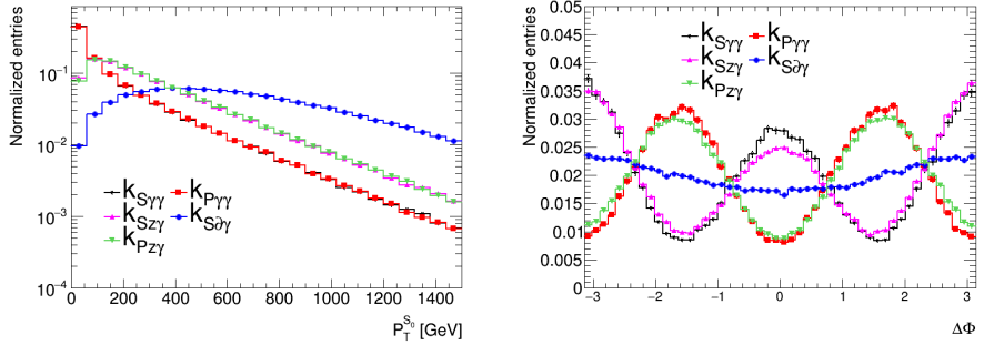
Рис. 7 — Распределение по поперечному импульсу гипотетического тяжёлого бозона Хиггса S_0 (слева) и по разнице азимутальных углов ассоциированных адронных струй в процессе pp \rightarrow S_0 jj \rightarrow \gamma\gamma jj (справа) [13].
