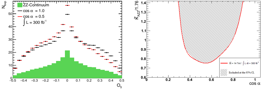
Рис. 4 — Пример распределения по специальной наблюдаемой O_5 , чувствительной к наличию смешанного CP-состояния бозона Хиггса (слева) и область исключения параметров модели на уровне интегральной светимости в 300 \text{fb}^{-1} (справа) [1].
