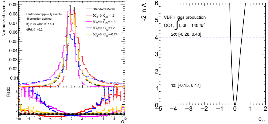
Рис. 6 — Распределение по оптимальной наблюдаемой OO_1 для процесса pp \rightarrow Hjj (слева) и результат сканирования функцией правдоподобия распределения по OO_1 в зависимости от величины константы связи c_{ZZ} (справа).
