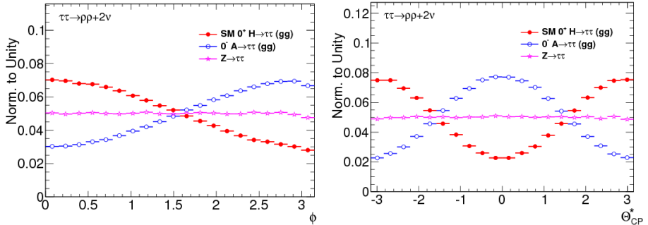
Рис. 5 — Распределения по угловым кинематическим переменным \phi (слева) и \Theta_{CP}^* (справа) для процесса pp \rightarrow H \rightarrow \tau\tau \rightarrow 2\rho 2\nu_\tau [3].
