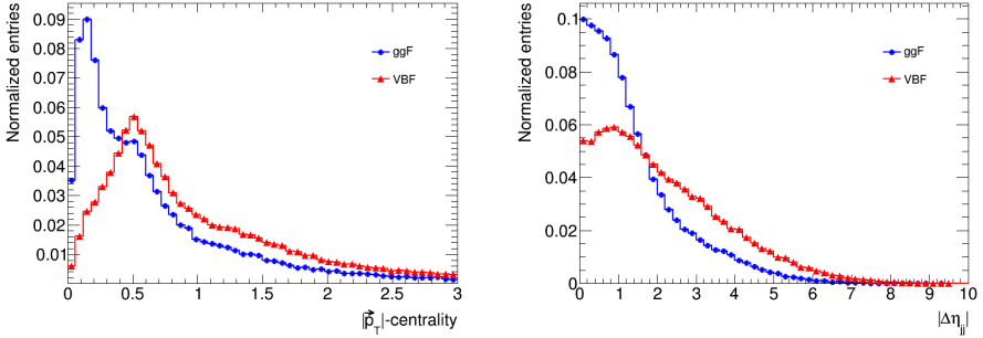
Рис. 8 — Распределение по p_T -центральности (слева) и абсолютной величине разности псевдобыстрот адронных струй (справа) в процессе pp \rightarrow Hjj для рождения бозона Хиггса с помощью механизмов ggF (синие маркеры) и VBF (красные маркеры), иллюстрирующие отличия в кинематике рассматриваемых механизмов рождения [8].
